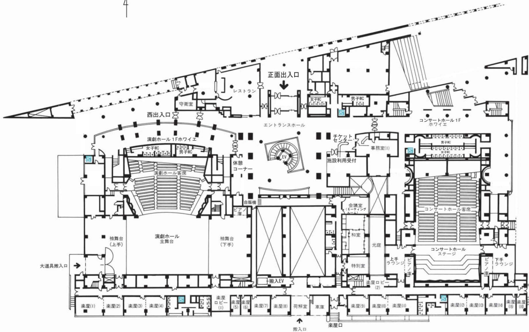
1階平面図 S=1:500
