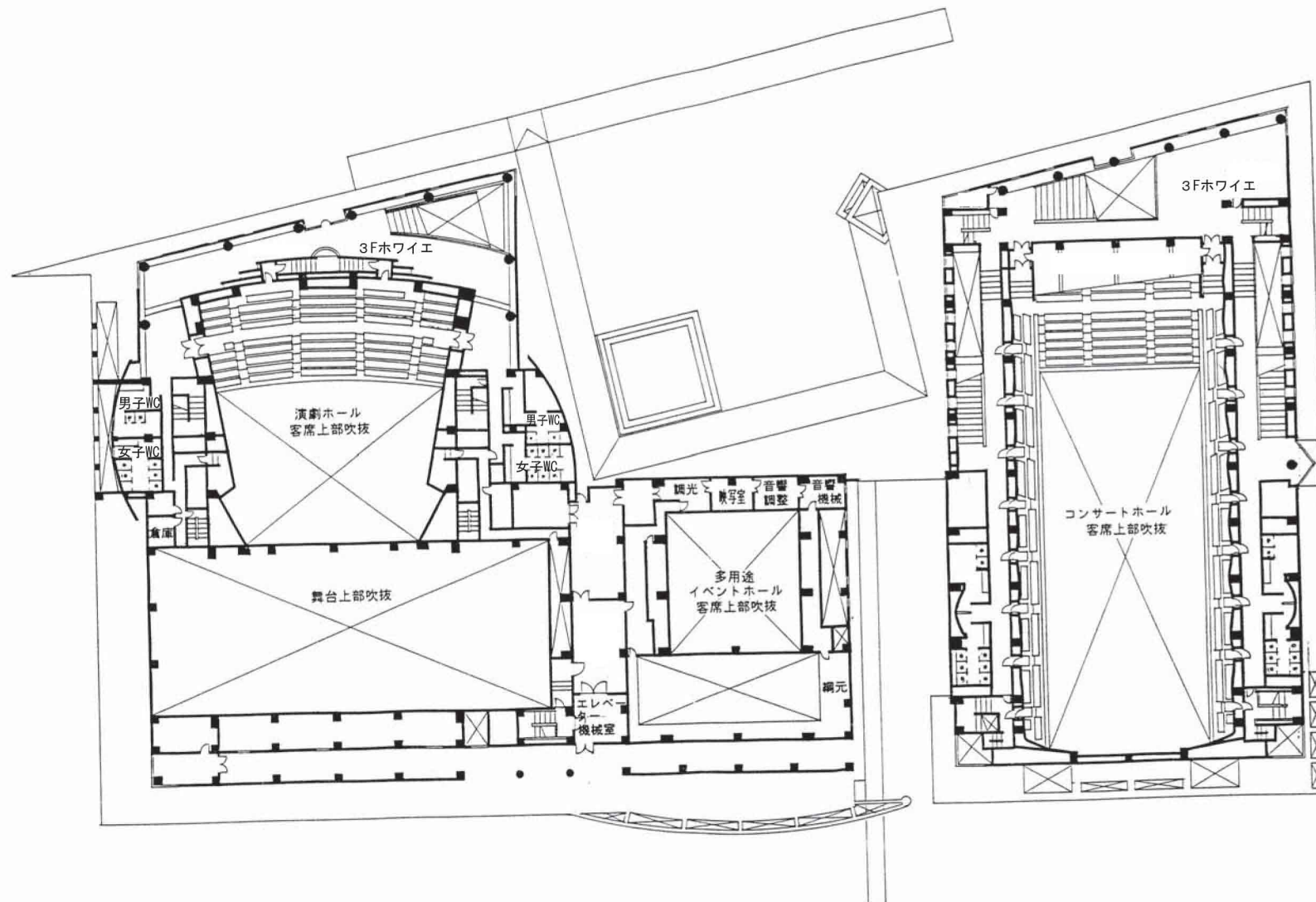
3階平面図 S = 1 : 500
